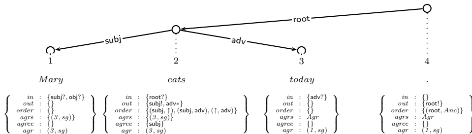
Abbildung 2.1: Dependenzgraph
